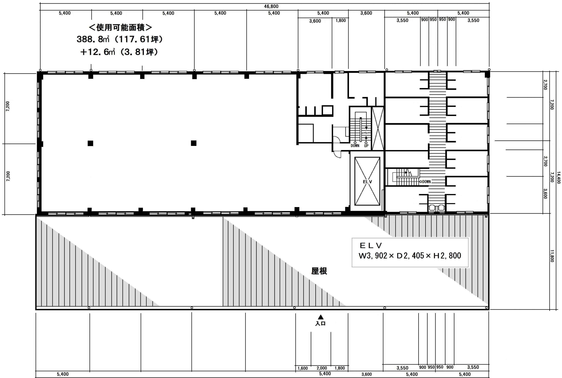
2F 平面図
